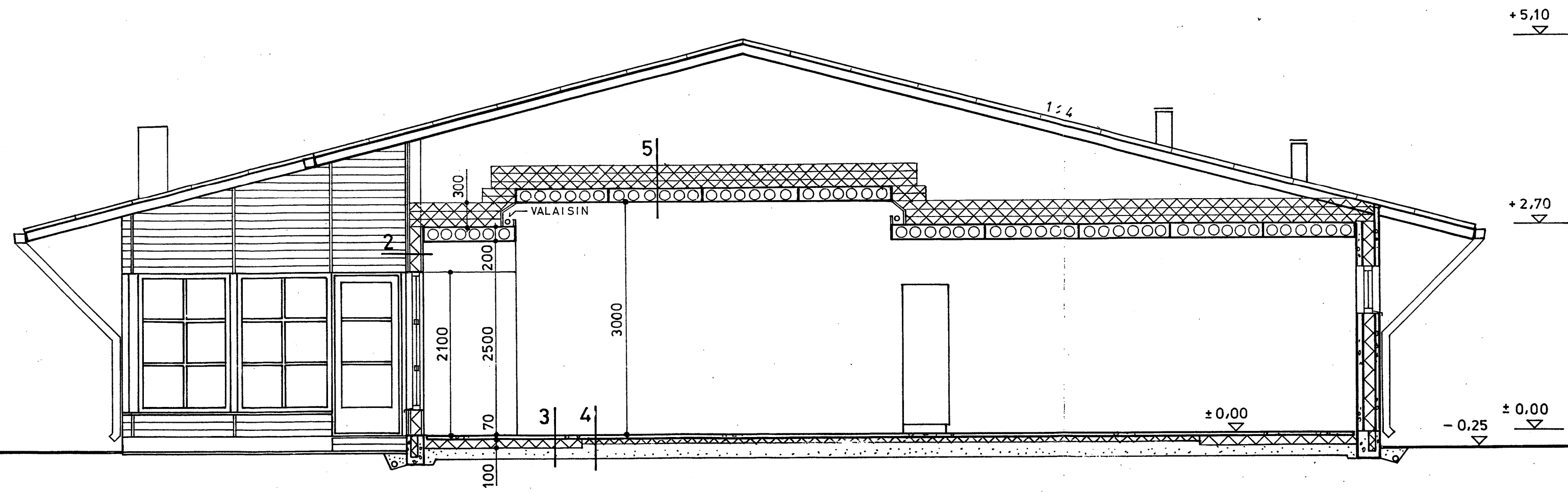
LEIKKAUS A - A
