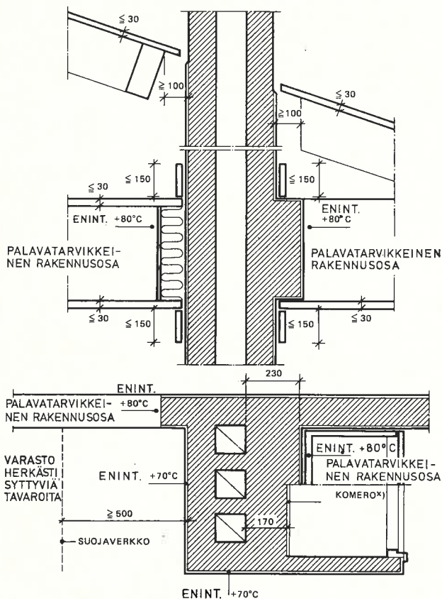
Kuva 5 I ryhmän tulisijan hormi
