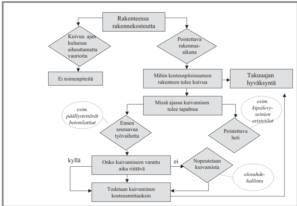
Kuva 5.2. Rakennekosteuden kuivatustarpeen ja kuivumisaika-arviointi /1/
