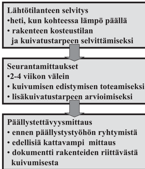
Kuva 5.4. Rakennekosteusmittausten kulku. Mittauksilla seurataan rakenteiden kuivumista ja varmistetaan riittävä kuivuminen.
