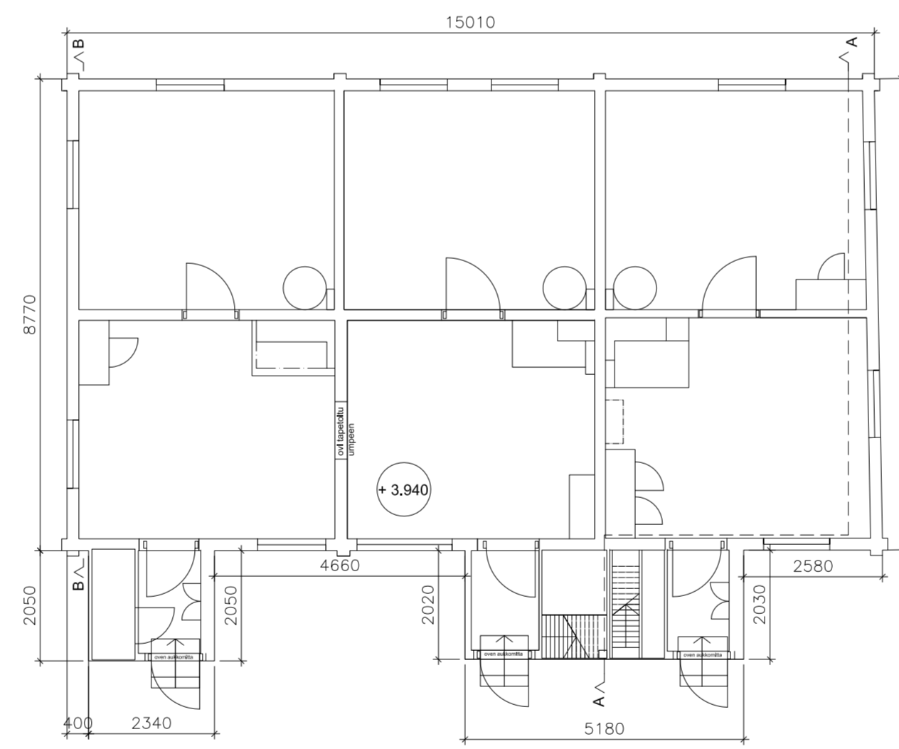
pohjapiirros 1:100
