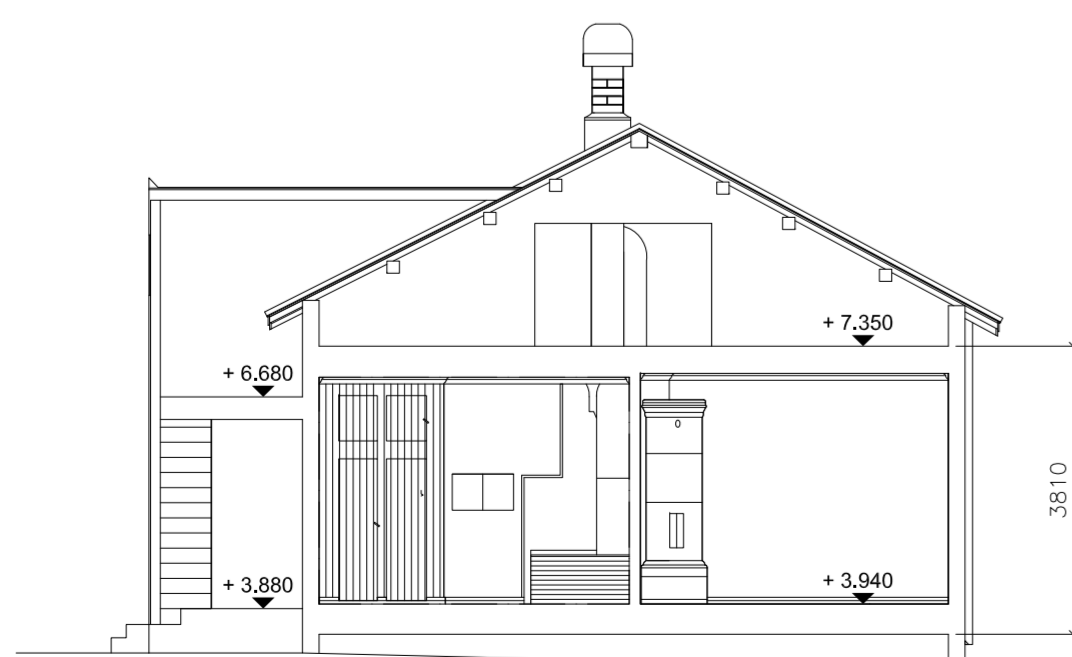
leikkaus A-A 1:100
