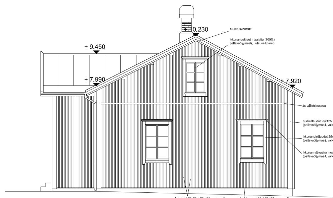
julkisivu lounaaseen 1:100
