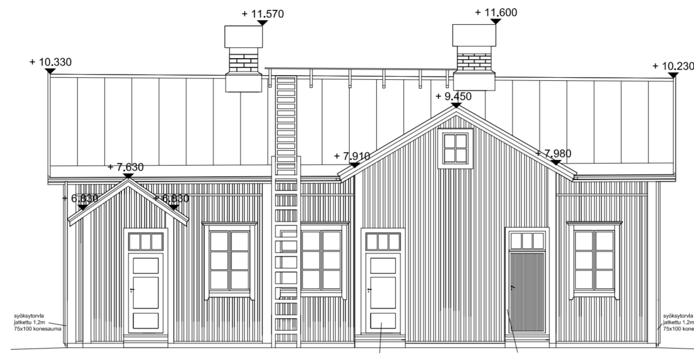
julkisivu luoteeseen 1:100
