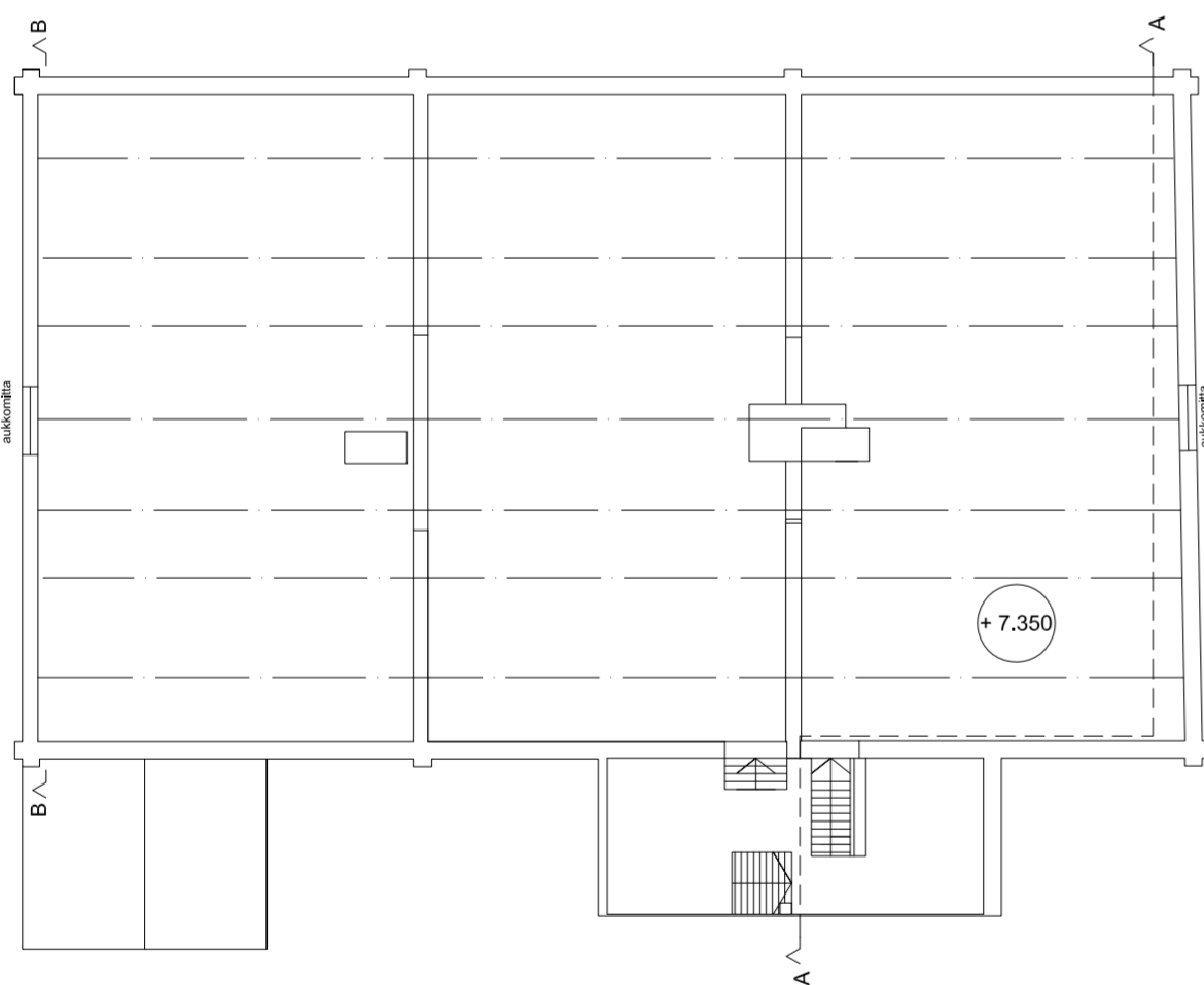
ullakko 1:100
