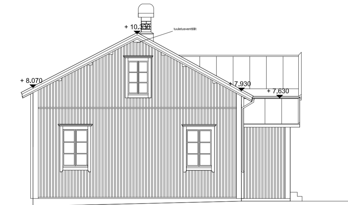
julkisivu koilliseen 1:100
