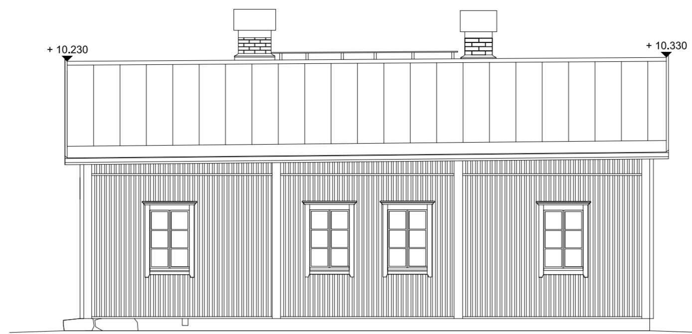
julkisivu kaakkoon 1:100
