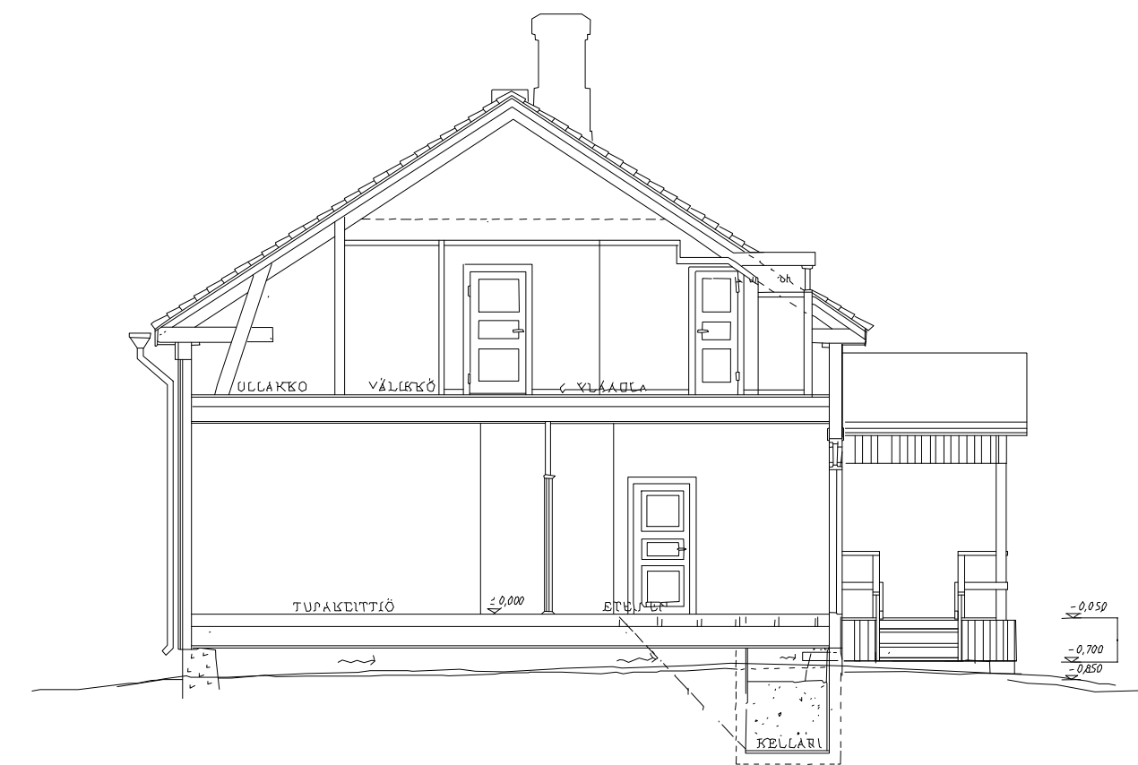
LEIKKAUS A-A
