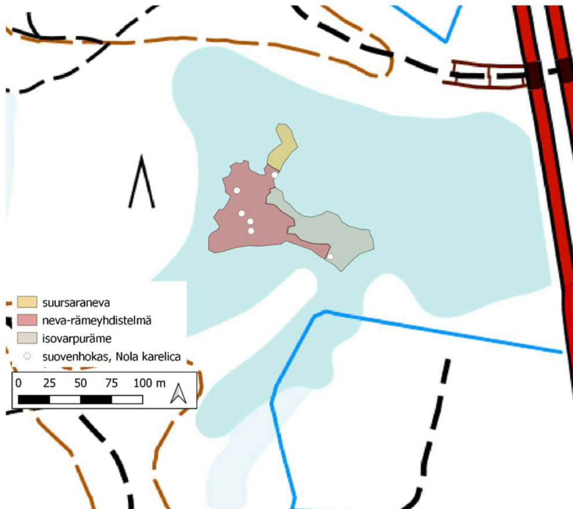
Kuva 3. Yleiskuva Ritaportin suunnittelualueen suotyypeistä ja suoventhokkaan aikuishavaintojen sijoittumisesta v. 2002.
