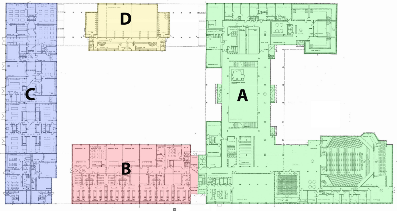
Pohjankartano muodostuu neljästä rakennusosasta, jotka muodostavat toiminnallisen kokonaisuuden. Julkisimmat toiminnot eli kirjasto, juhlasali ja luentosali (osa A) sijoittuvat päälähestymissuuntaan, etupihaa suojaamaan.
