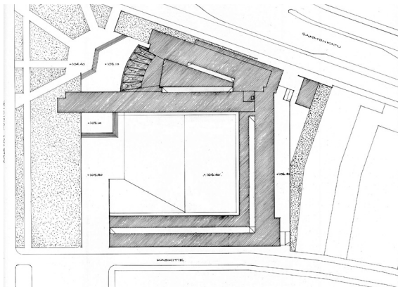
Kari Virran ja Timo Penttilän suunnittelemassa Tampereen Sampolan työväenopiston ja kansalaiskoulun rakennuksessa on samoja typologisia piirteitä kuin Pohjankartanossa. (Arkkitehti 10/1962, 205, 209)
