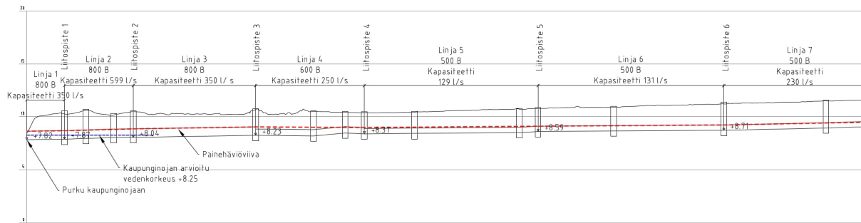
Kuva 13. Painehäviölaskennan tulos pituusleikkauksessa linjalla A-A liittospisteet 1-6
