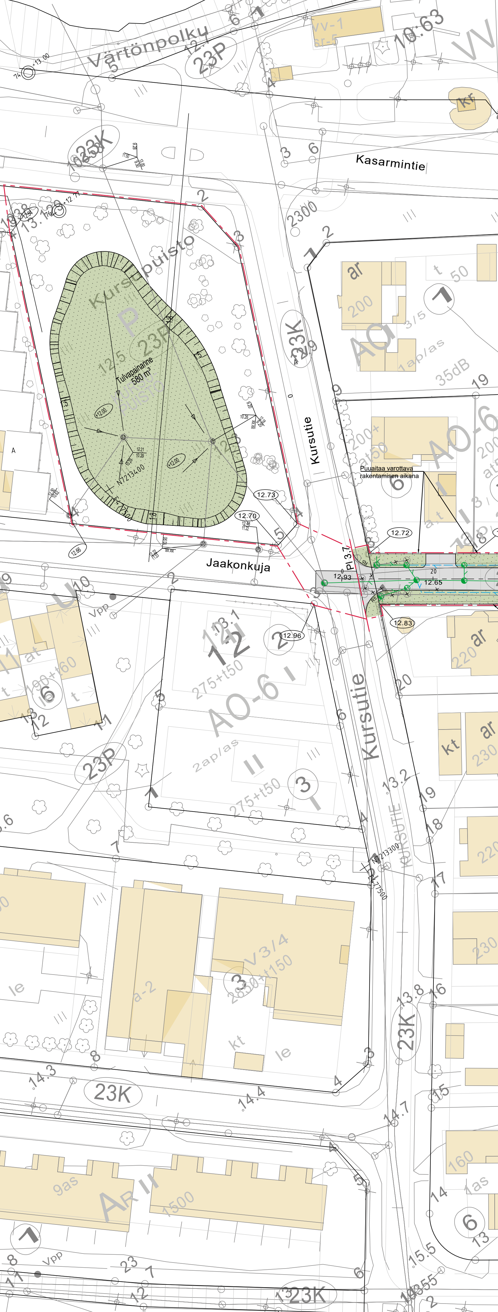
SUUNNITELMAKARTTA 1:500
