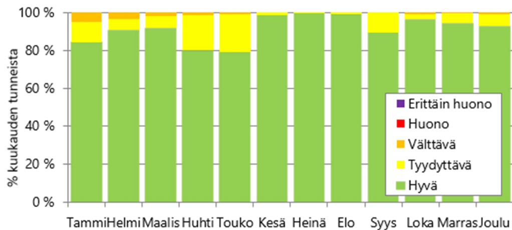
Kuvio 26. Ilmanlaadun jakautuminen eri ilmanlaatuiluokkiin kuukausittain Pyykösjärvellä vuonna 2024.
