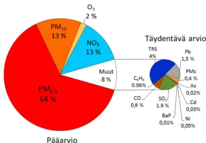
Kuva 10. Ilman epäpuhtauksien Suomessa vuonna 2013 aiheuttaman tautitaakan jakautuminen eri epäpuhtauksien kesken. TRS= pelkistyneet rikkiyhdisteet, C_6H_6 =bentseeni, PMc = karkeat hiukkaset (Ympäristöministeriö 2016).
