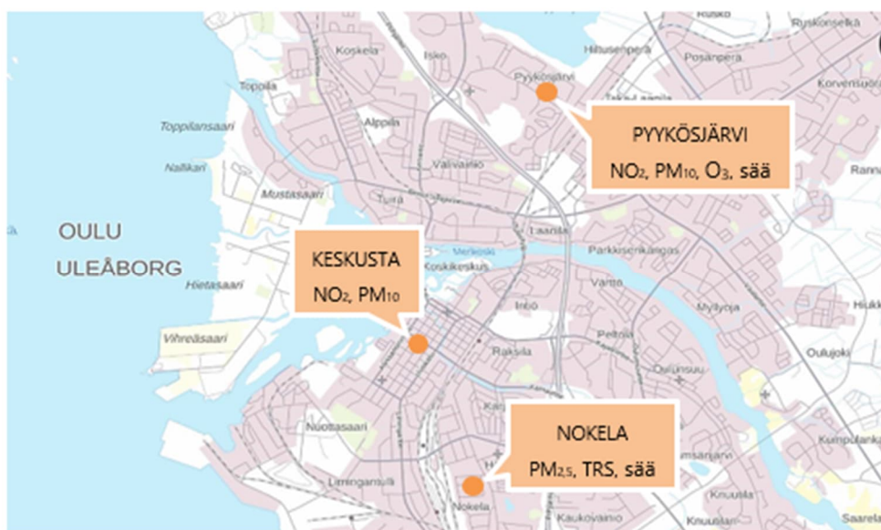
Kuva 1. Oulun ilmanlaadun mittausasemien sijainti ja mitattavat suureet vuonna 2024.
