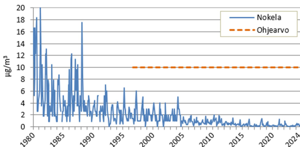
Kuvio 24. TRS-yhdisteiden ohjearvoon verrannollisten kuukauden 2. korkeimpien vuorokausiarvojen kehitys Nokelassa vuosina 1980-2024.
