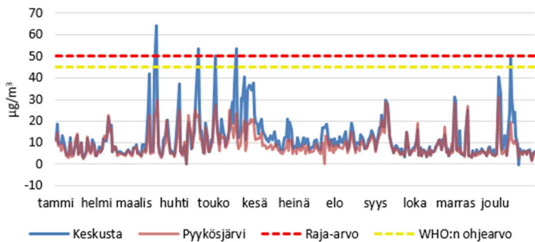
Kuvio 5. Hengitettävien hiukkasten vuorokausiarvot Keskustassa ja Pyykösjärvellä vuonna 2024.
