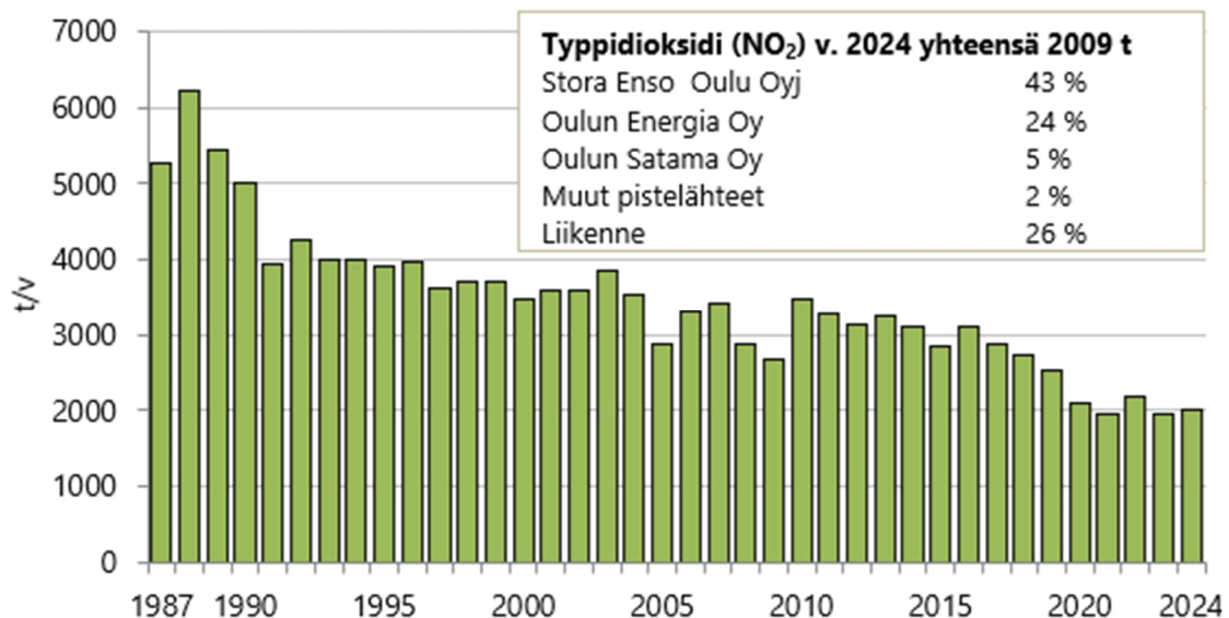
Kuvio 27. Yhteenlasketut typpidioksidipäästöt (NO 2 ) Oulussa vuosina 1987–2024 ja niiden jakautuminen päästölähteittäin.
