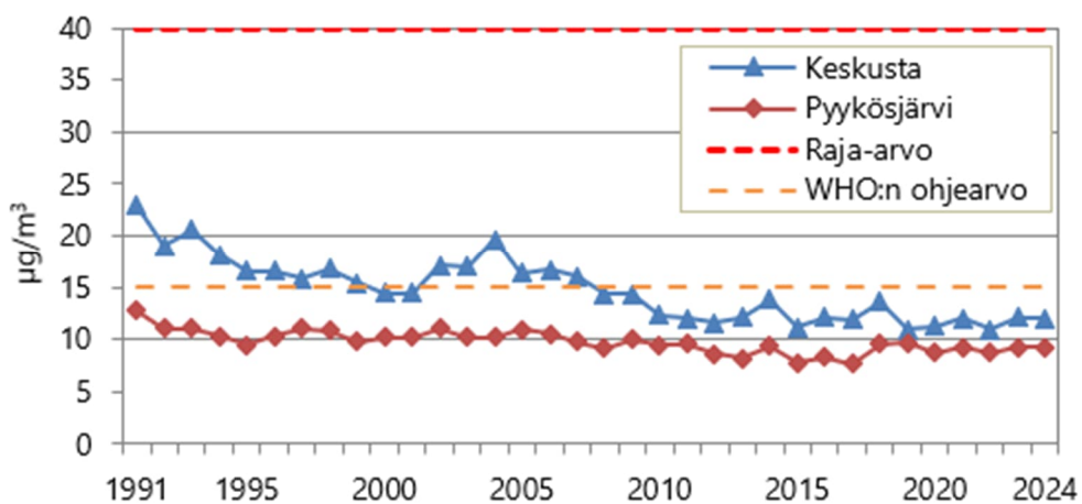
Kuvio 6. Hengitettävien hiukkasten vuosikeskiarvojen kehitys vuosina 1991-2024.
