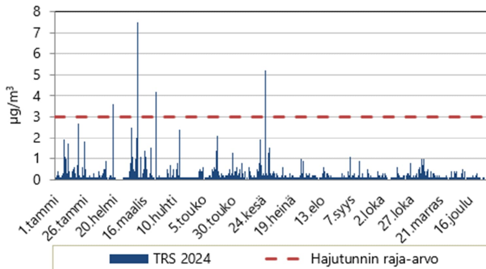
Kuvio 22. TRS-yhdisteiden tuntipitoisuudet vuonna 2024.
