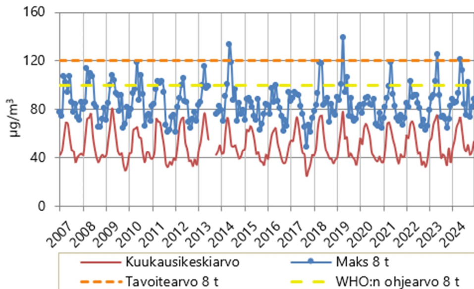
Kuvio 21. Otsonin kuukausikeskiarvot ja kuukauden korkeimmat 8 tunnin keskiarvot vuosina 2007–2024.
