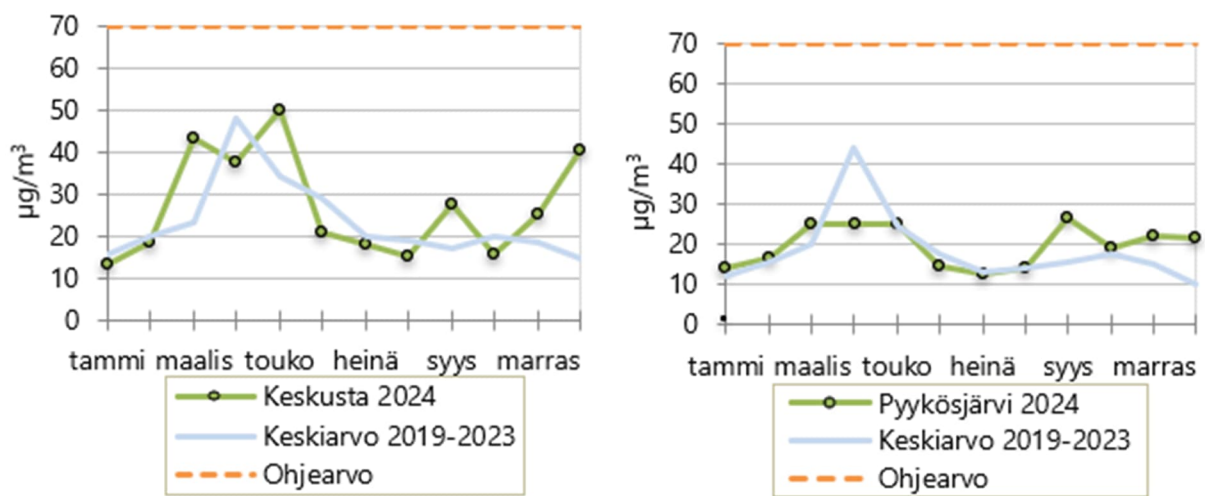
Kuvio 7. ja 8. Hengitettävien hiukkasten ohjearvoon verrannolliset kuukauden 2. korkeimmat vuorokausiarvot ja niiden keskiarvo vuosina 2019-2023 Keskustassa (vasen) ja Pyykösjärvellä (oikea).
