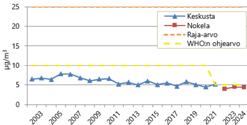
Kuvio 10. Pienhiukkasten vuosikeskiarvojen kehitys vuosina 2002–2021 Keskustassa ja vuosina 2022–2024 Nokelassa.
