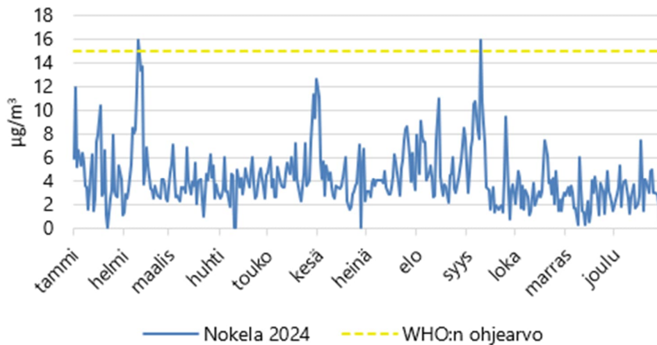
Kuvio 11. Pienhiukkasten vuorokausiarvot Nokelassa vuonna 2024.
