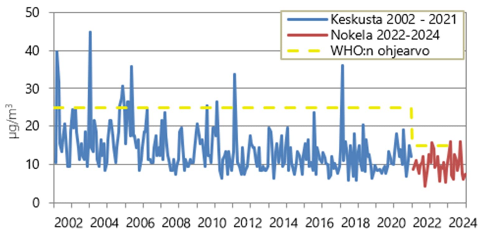
Kuvio 12. Pienhiukkasten kuukauden korkeimmat vuorokausiarvot Keskustassa vuosina 2002-2021 ja Nokelassa vuosina 2022-2024.
