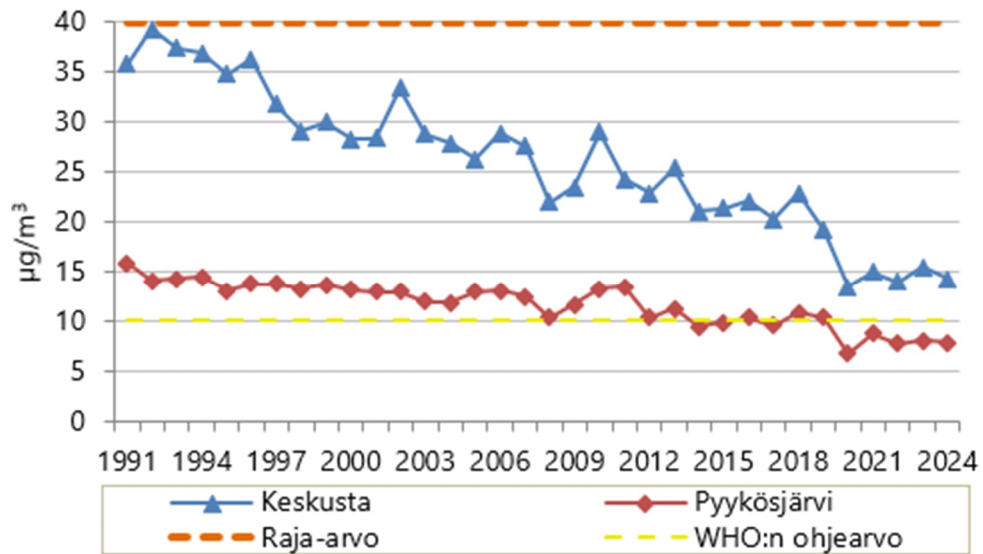
Kuvio 15. Typpidioksidin vuosikeskiarvojen kehitys vuodesta 1991 vuoteen 2024 Keskustassa ja Pyykösjärvellä.
