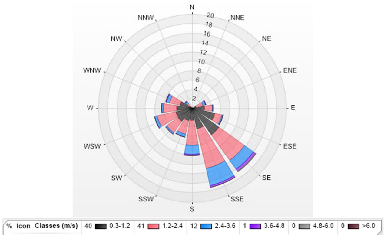
Kuvio 3. Tuulen suuntien osuudet ja tuulen nopeuden jakautuminen eri nopeusluokkiin tuulensuunnittain vuonna 2024 Pyykösjärven mittausasemalla.
