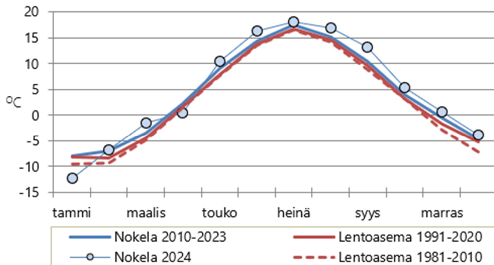
Kuvio 1. Kuukauden keskilämpötilat Nokelassa vuonna 2024 sekä vuosien 2010-2023 keskiarvo Nokelassa ja vertailujaksoilla vuosina 1991-2020 ja 1981-2010 Oulunsalon lentoasemalla.
