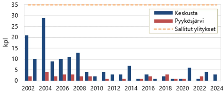
Kuvio 4. Hengitettävien hiukkasten vuorokausiraja-arvon 50 \mu\text{g}/\text{m}^3 ylitysten lukumäärä Keskustassa ja Pyykösjärvellä vuosina 2002-2024.
