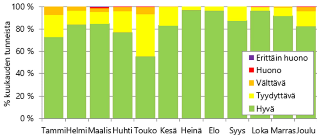
Kuvio 25. Ilmanlaadun jakautuminen eri ilmanlaatuiluokkiin kuukausittain Oulun keskustassa vuonna 2024.
