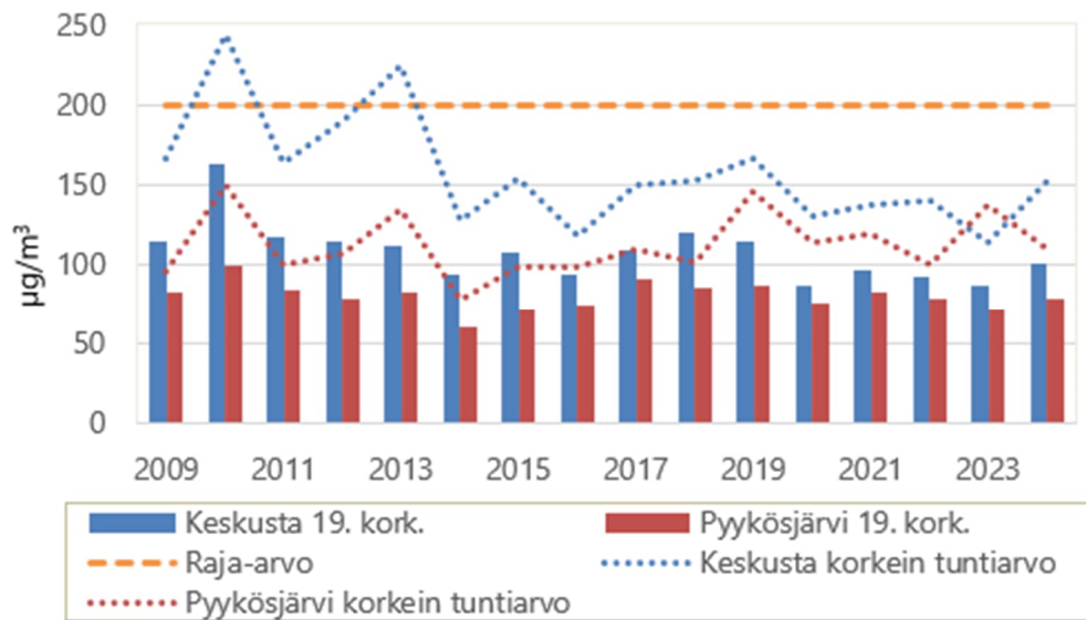
Kuvio 13. Typpidioksidin raja-arvoon verrannolliset 19. korkeimmat sekä korkeimmat tuntiarvot vuosina 2009–2024 Keskustassa ja Pyykösjärvellä.
