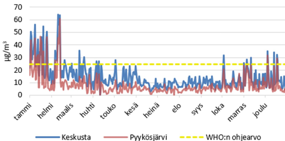
Kuvio 16. Typpidioksidin vuorokausiarvot Keskustassa ja Pyykösjärvellä vuonna 2024.
