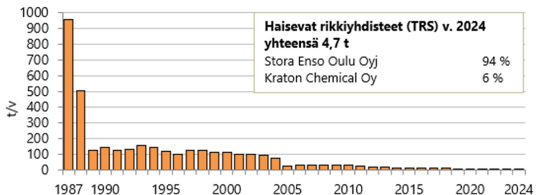
Kuvio 30. Yhteenlasketut haisevien rikkiyhdisteiden (TRS) päästöt Oulussa vuosina 1987-2024 ja niiden jakautuminen päästölähteittäin.
