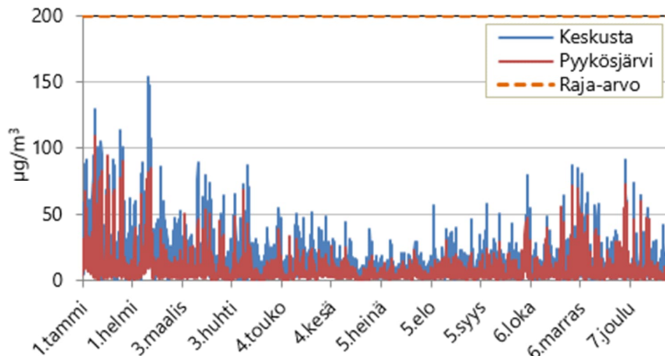
Kuvio 14. Typpidioksidin tuntiarvot vuonna 2024 Keskustassa ja Pyykösjärvellä.
