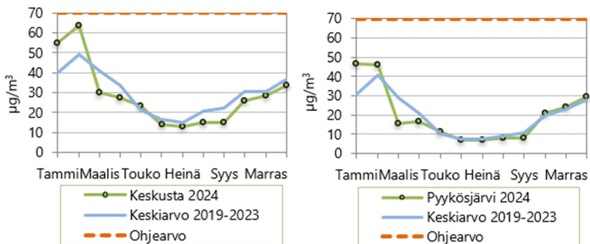
Kuvio 19. ja 20. Typidioksidin vuorokausiohjearvoon verrannolliset kuukauden 2. korkeimmat vuorokausiarvot vuonna 2024 ja niiden keskiarvot vuosina 2019-2023 Keskustassa (vasen) ja Pyykösjärvellä (oikea).
