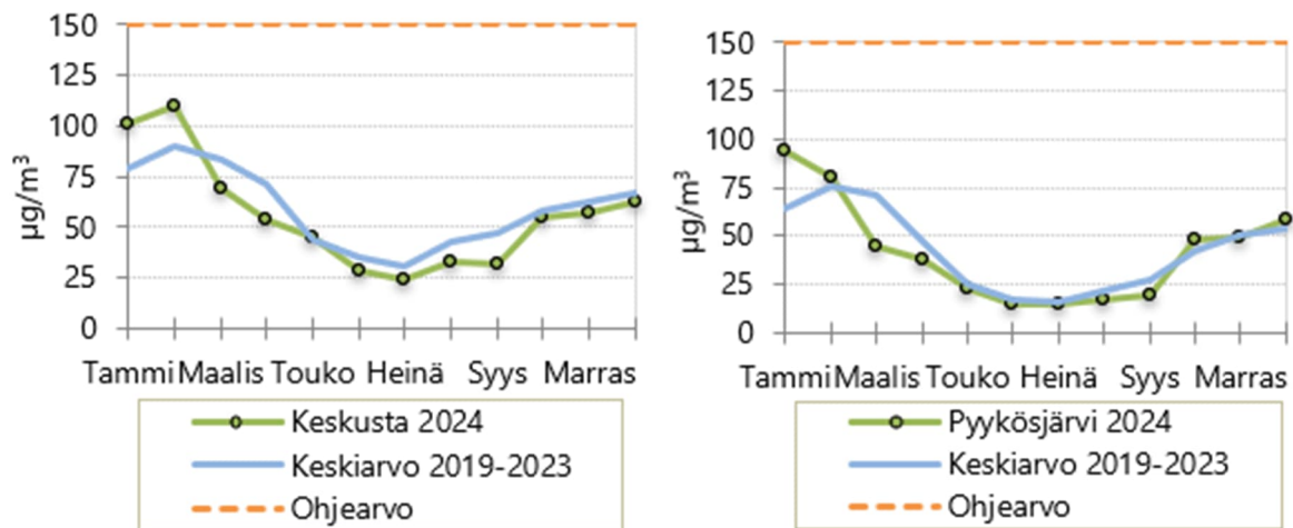
Kuvio 17. ja 18. Typidioksidin tuntiohjearvoon verrannolliset 99.prosenttipisteen tuntipitoisuudet vuonna 2024 ja niiden keskiarvot vuosina 2019-2023 Keskustassa (vasen) ja Pyykösjärvellä (oikea).
