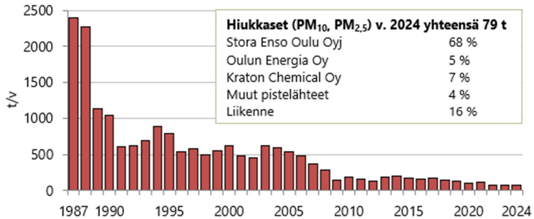
Kuvio 28. Yhteenlasketut hiukkaspäästöt (PM 10 , PM 2,5 ) Oulussa vuosina 1987-2024 ja niiden jakautuminen päästölähteittäin.
