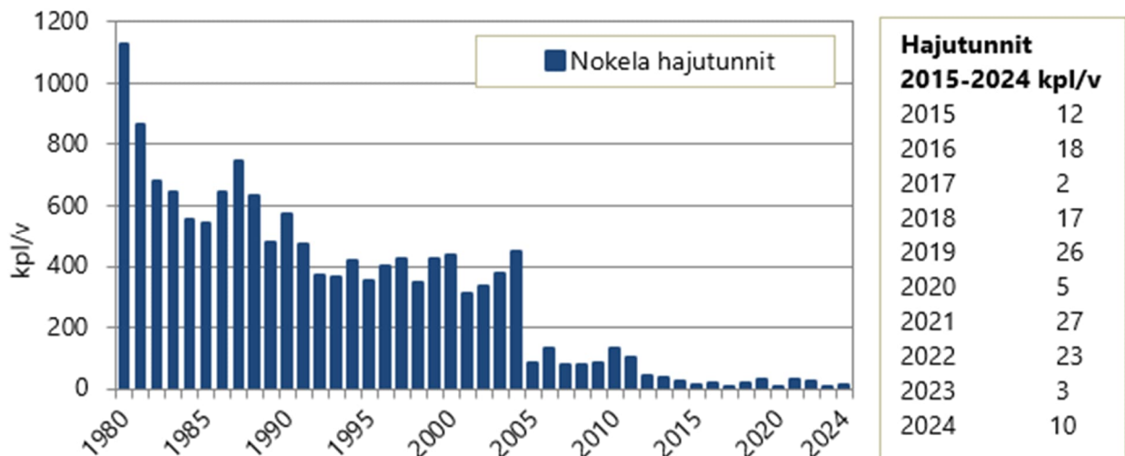
Kuvio 23. TRS-yhdisteiden hajutuntien määrä vuosittain Nokelassa vuosina 1980-2024.
