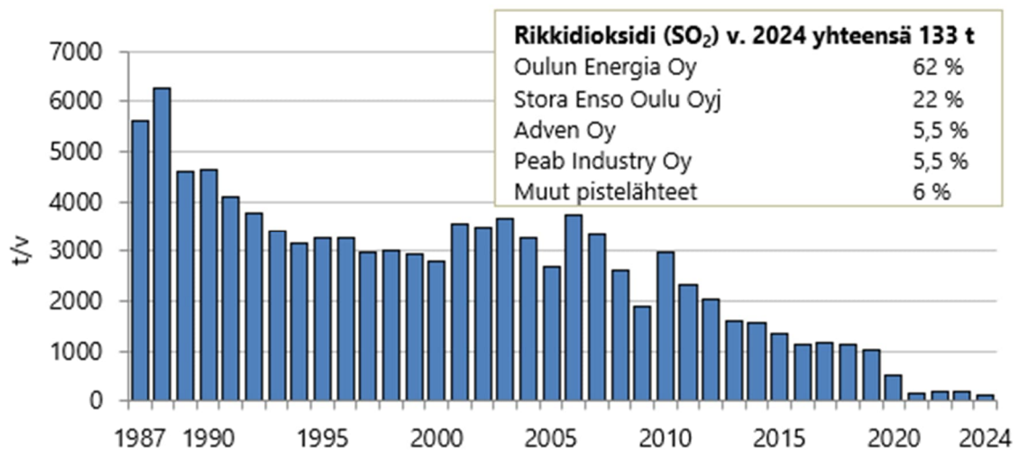
Kuvio 29. Yhteenlasketut rikkidioksidipäästöt (SO 2 ) Oulussa vuosina 1987-2024 ja niiden jakautuminen päästölähteittäin.
