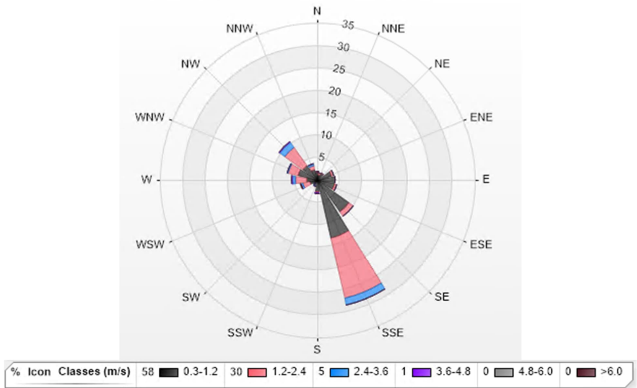
Kuvio 2. Tuulen suuntien osuudet ja tuulen nopeuden jakautuminen eri nopeusluokkiin tuulensuunnittain vuonna 2024 Nokelan mittausasemalla.
