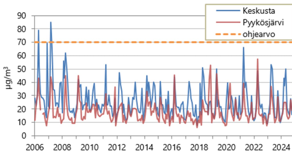
Kuvio 9. Hengitettävien hiukkasten ohjearvoon verrannollisten kuukauden 2. korkeimpien vuorokausiarvojen kehitys vuosina 2006-2024 Keskustassa ja Pyykösjärvellä.
