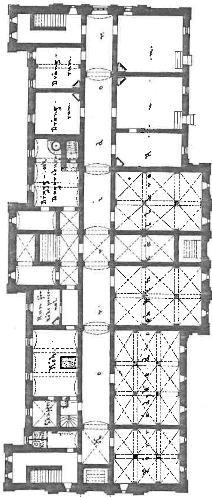
Plan af källarvåningen.
