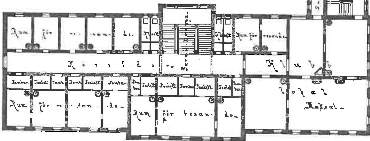
Plan af 1 de våningen
