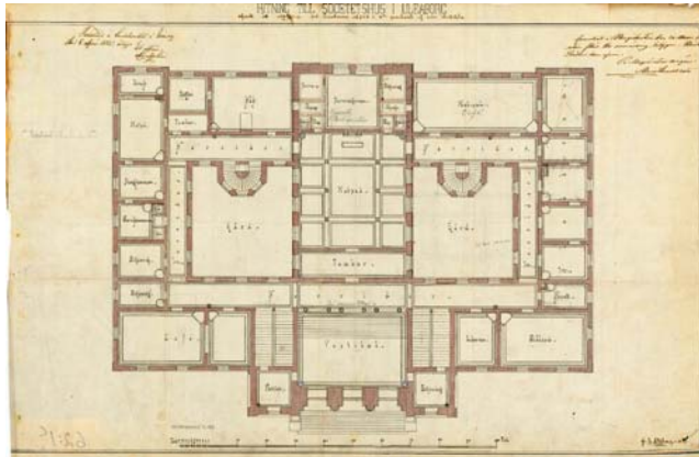
Pohjapiirustus 1, krs. J.E. Stenberg (1885).
