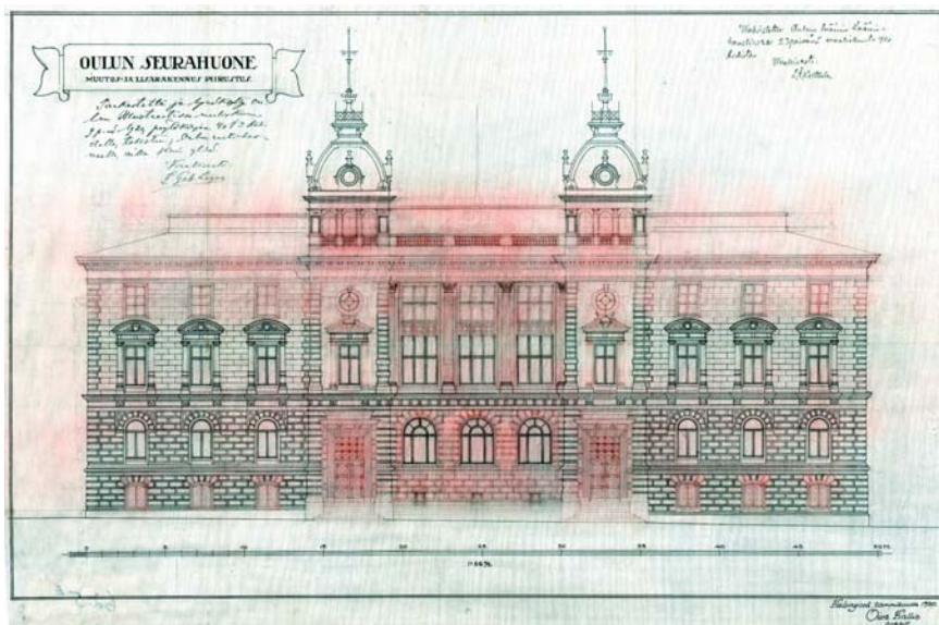
Julkisivu Kirkkokadulle. Oiva Kallion muutospiirustus v. 1920.
