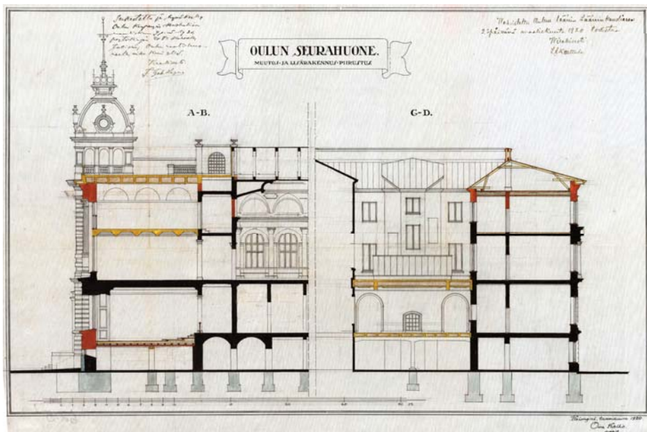
Leikkauspiirustus. Oiva Kallio, v. 1920.
