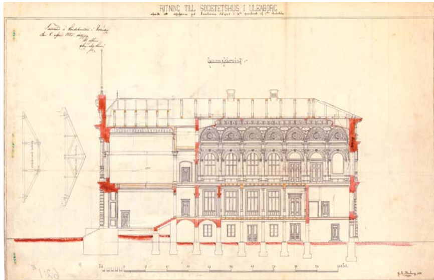
Leikkauspiirustus juhlasalin kohdalta. J. E. Stenberg, 1885.
