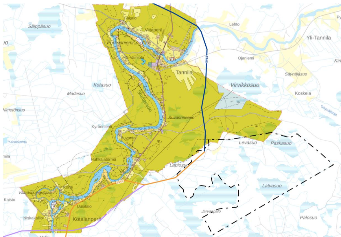
Kuva 6. Suunnittelualueen raja ja suunnitellut voimajohtolinjat suhteessa Suurajoen osayleiskaavaan.
