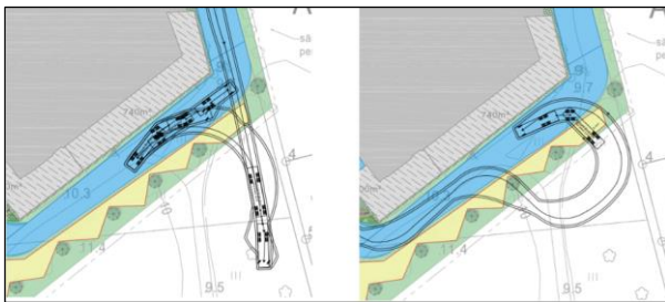
Kuva 26. Tilantarve Kollaanpuistossa, jos Musiikkikeskuksen tavarankuljetuksen täysperävaunuyhdistelmä kääntyisi ilman rakennuksen ympäriajomahdollisuutta (saapuminen Ketokadun suunnasta ja Leevi Madetojan kadun suunnasta).
