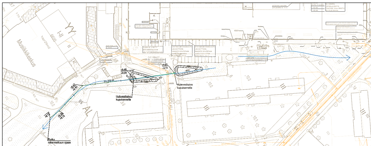
Kuva 21. Alueellisen tulvareitin kulkureitit tonttien itäosassa (siniset nuolet). (Ramboll Finland Oy, 16.4.2022)
