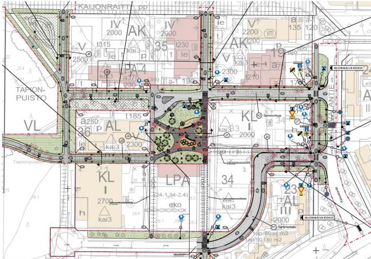
Kuva 19. Ote katusuunnitelmasta (Sitowise Oy 2024).
