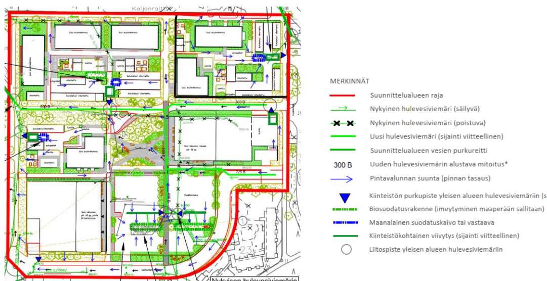
Kuva 17. Ote hulevesisuunnitelmasta (Sitowise Oy 2023).
