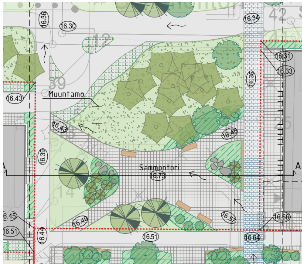
Kuva 18. Ote ympäristön yleissuunnitelmasta (Sitowise 2023).
