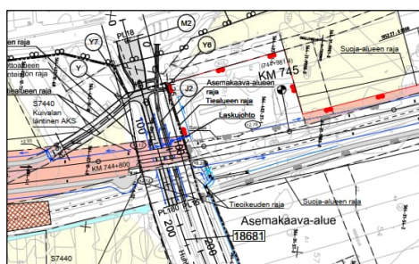
Kuvat 7 ja 8. Ote ratasuunnitelmasta Perävainion kohdalta. Ylempi Porttiväylän ja Visiipuiston ja alempi Maaniitynpuiston ja Huhtakalliontien alikulun kohdalta. (Kmv 744+800 – 745+800).
