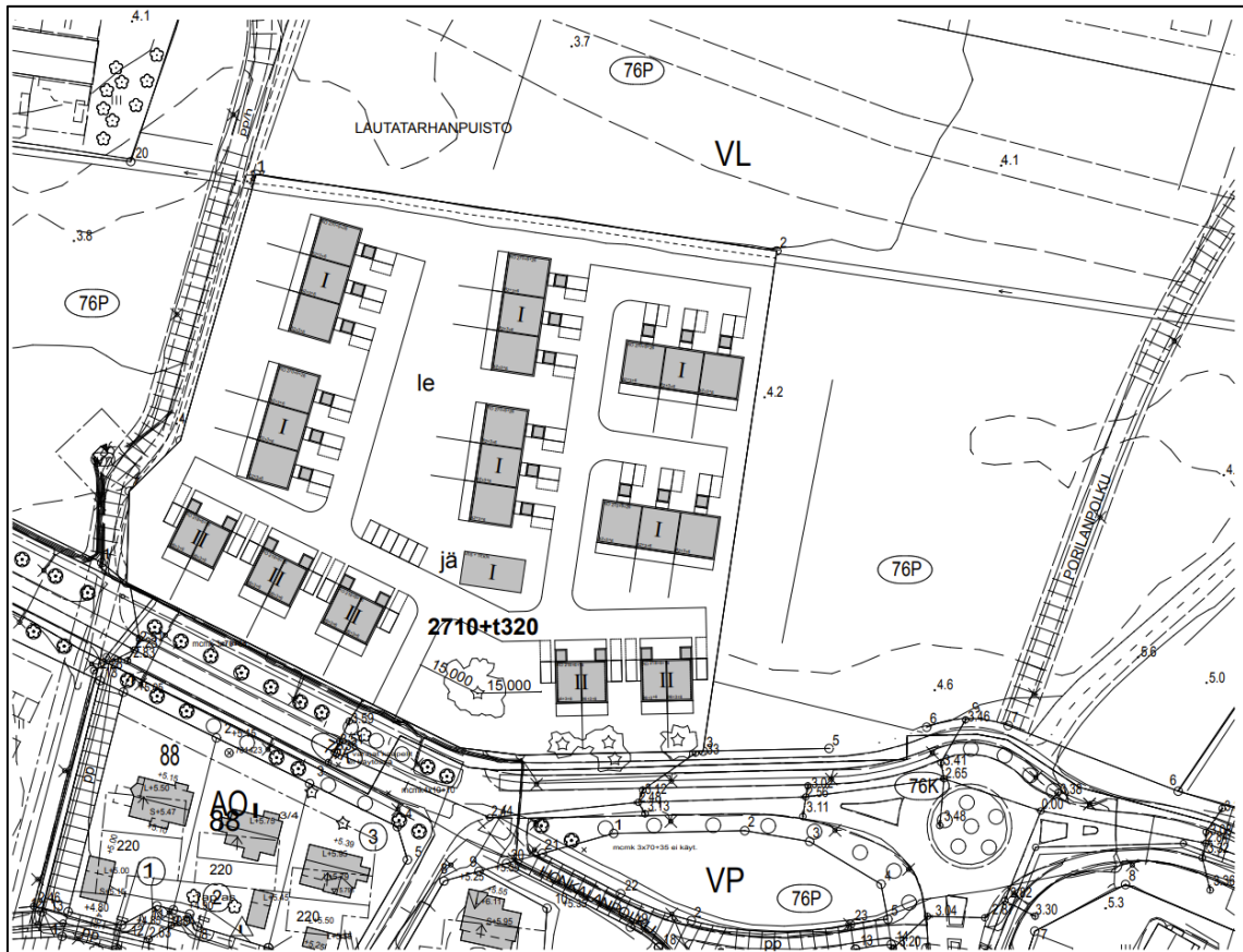
Kuva 1-1. Kiinteistön 564-76-223-1 asemapiirros (Arkkitehtitoimisto Veli Karjalainen Oy 7.8.2024).
