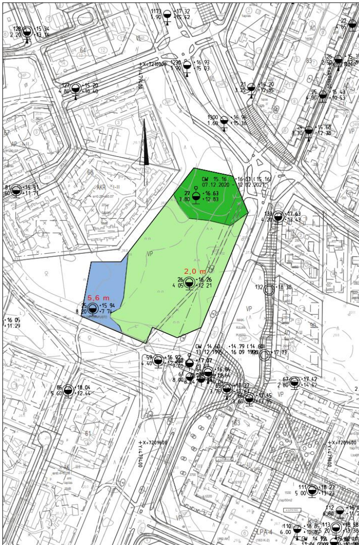
Kuva 11. Maikkulantien rakennettavuuskartta.
