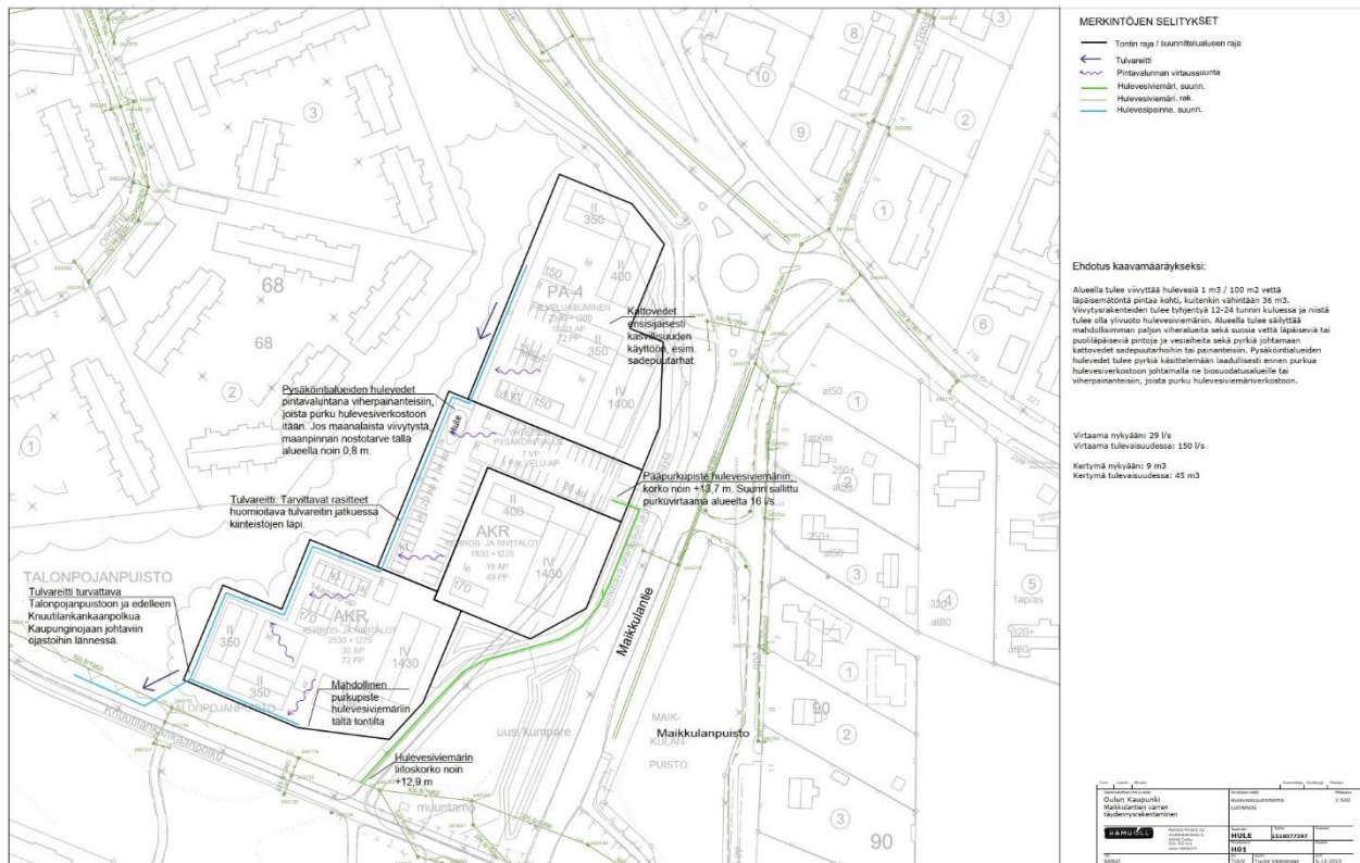
Kuva 26. Maikkulantien varren hulevesisuunnitelma. Lähde: Ramboll Finland Oy, 2023.
