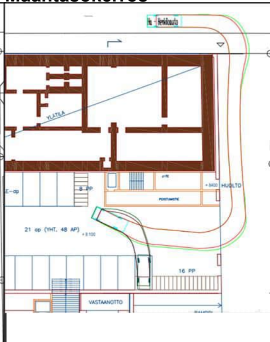
Kuva 15. Ajourat kellar- ja maantasokerrokseen (henkilöauto).
