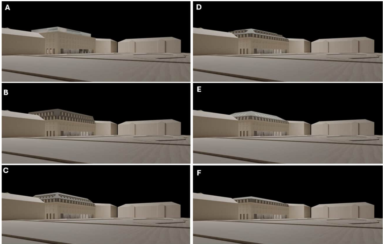
Kuva 29 Kaavaluonnosvaiheen jälkeen tutkittuja erilaisia kattomaailman massoitteluja, näkymät maantasosta. Kuvat: JKMM Arkkitehdit Oy.
