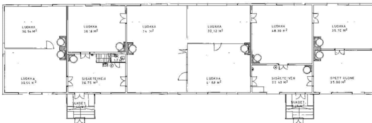
Kuva 13 Alkuperäinen pohjapiirustus.
