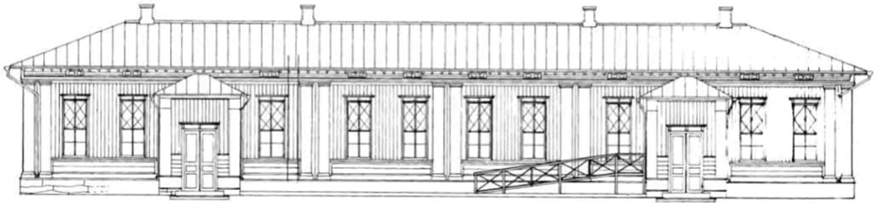
Kuva 15 Ote rakennushistoria selvityksestä, pääpiirustuskuva pohjoisjulkisivusta 20.12.1977. Esteetön sisäänkäynti rakennettiin länsipäädyn puoleiseen kuistiin vuoden 1979 perusparannuksen yhteydessä.
