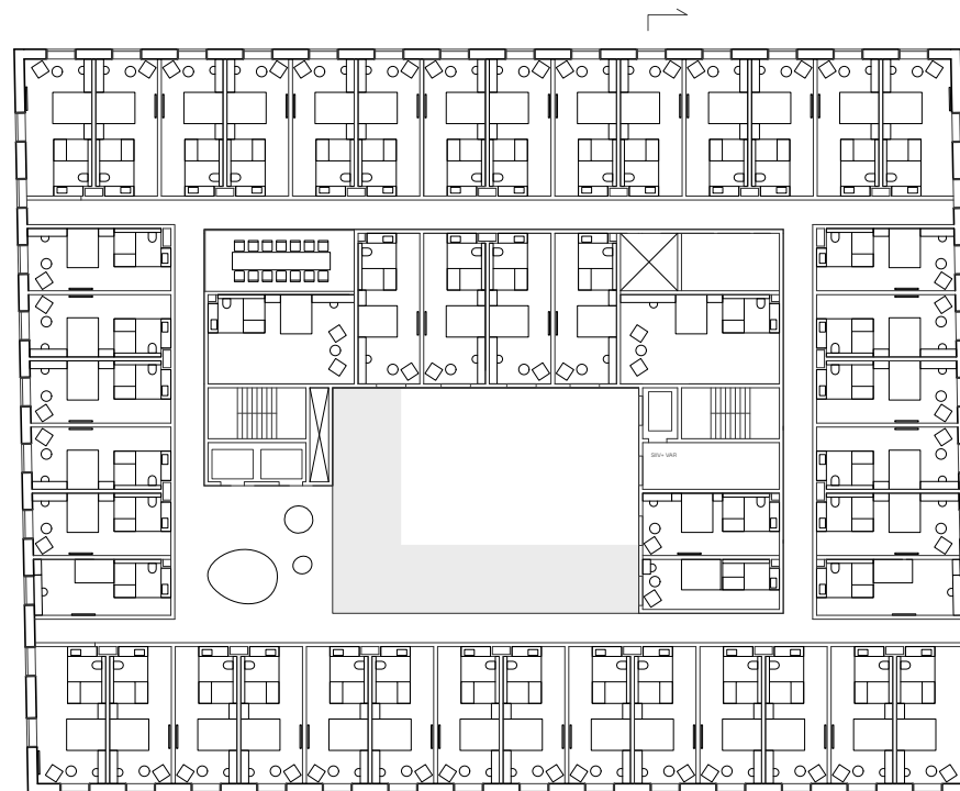
HOTELLI KERROS 48 HUONETTA
