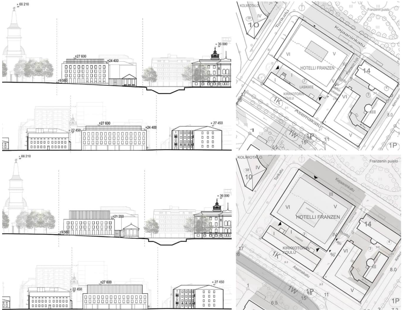
Kuva 31 Kuvavertailu, aluejulkisivut ja asemapiirrokset. Ylemmät kuvat: asemakaavan muutosluonnosvaiheen viitesuunnitelmat 5.6.2025. Alemmat kuvat: Asemakaavan muutosehdotusvaiheen viitesuunnitelmat 19.12.2025. Kuvat: JKMM Arkkitehdit Oy.
