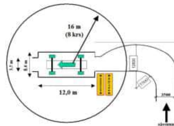
Kuva 24. Tikasauton ulottuma 8.krs asti tikasauton keskeltä mitattuna sekä tassulevityspaikan koko (Pohjois-Pohjanmaan pelastuslaitos 2024).
