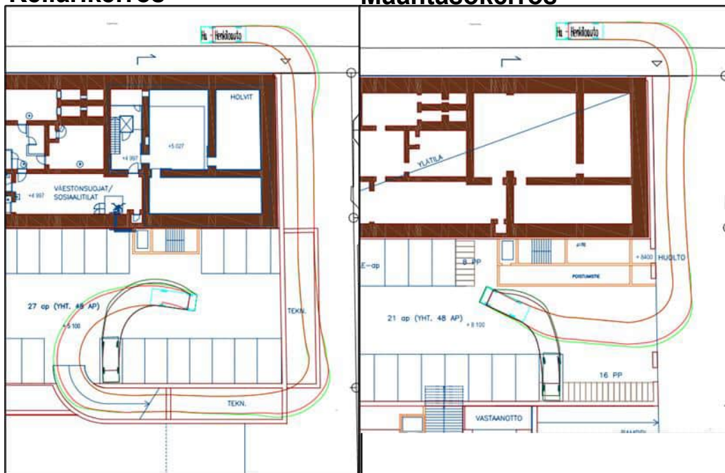
Kuva 15. Ajourat kellar- ja maantasokerrokseen (henkilöauto).
