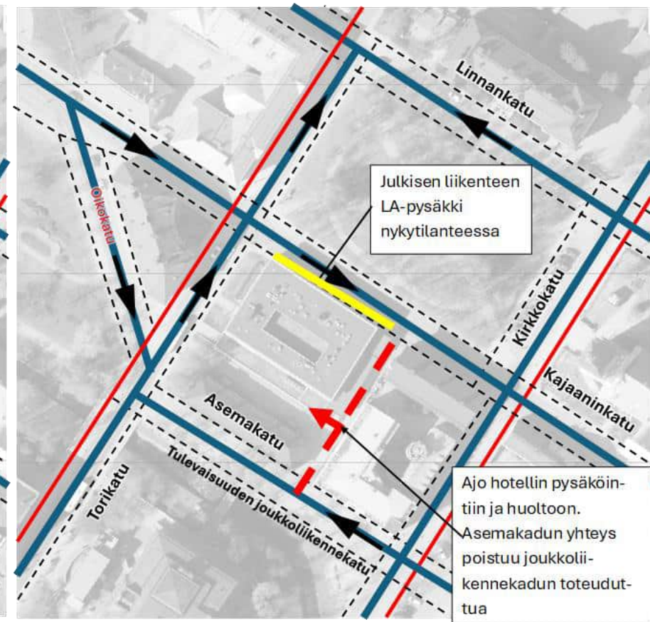
Kuva 22. Liikennekaavio tavoitetilanteessa.
