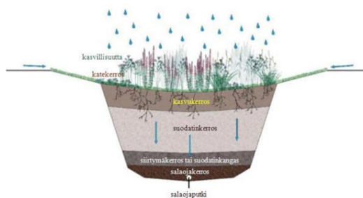
Kuva 14. Biosuodatuksen tyyppirakenne ( Hulevesien hallintarakenteet ja niiden kunnossapito, Ilmastokestävä kaupunki ).
