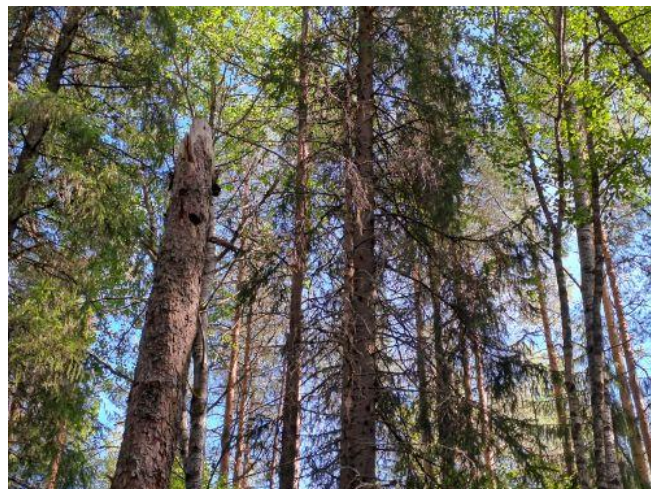
Kuvio 15. Kuvat 17 ja 18. Komeaa varttunutta tuoretta kangasta, jolla paikoin reilusti maalahopuuta. Paikoin myös mäntykeloja ja lehtipuupökölöitä.
