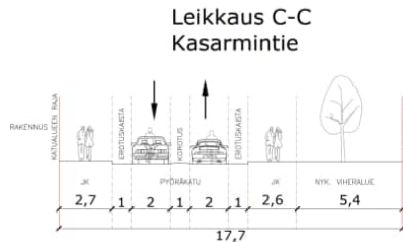
Kuva 8. Kasarmintien poikkileikkaus
