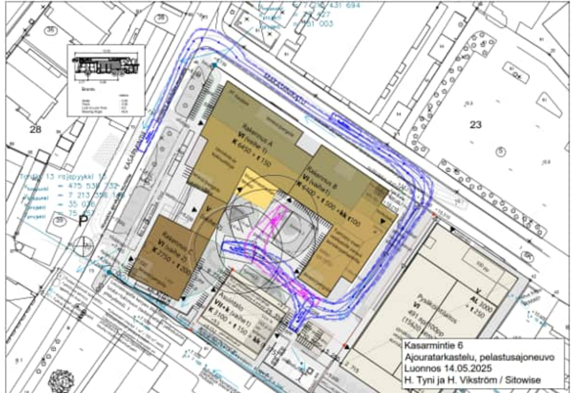
Kuva 24. Huoltoajoneuvojen ajourat
