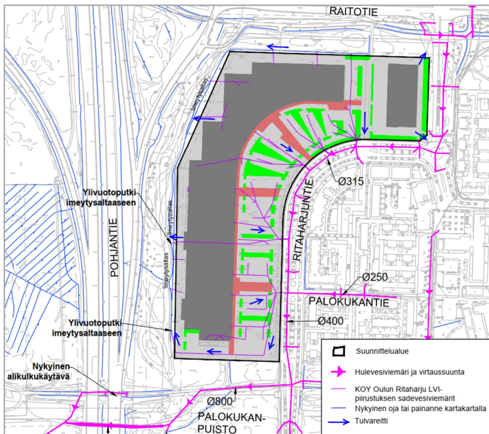
Kuva 8. Suunnittelualueen nykyinen hulevesijärjestelmä.
