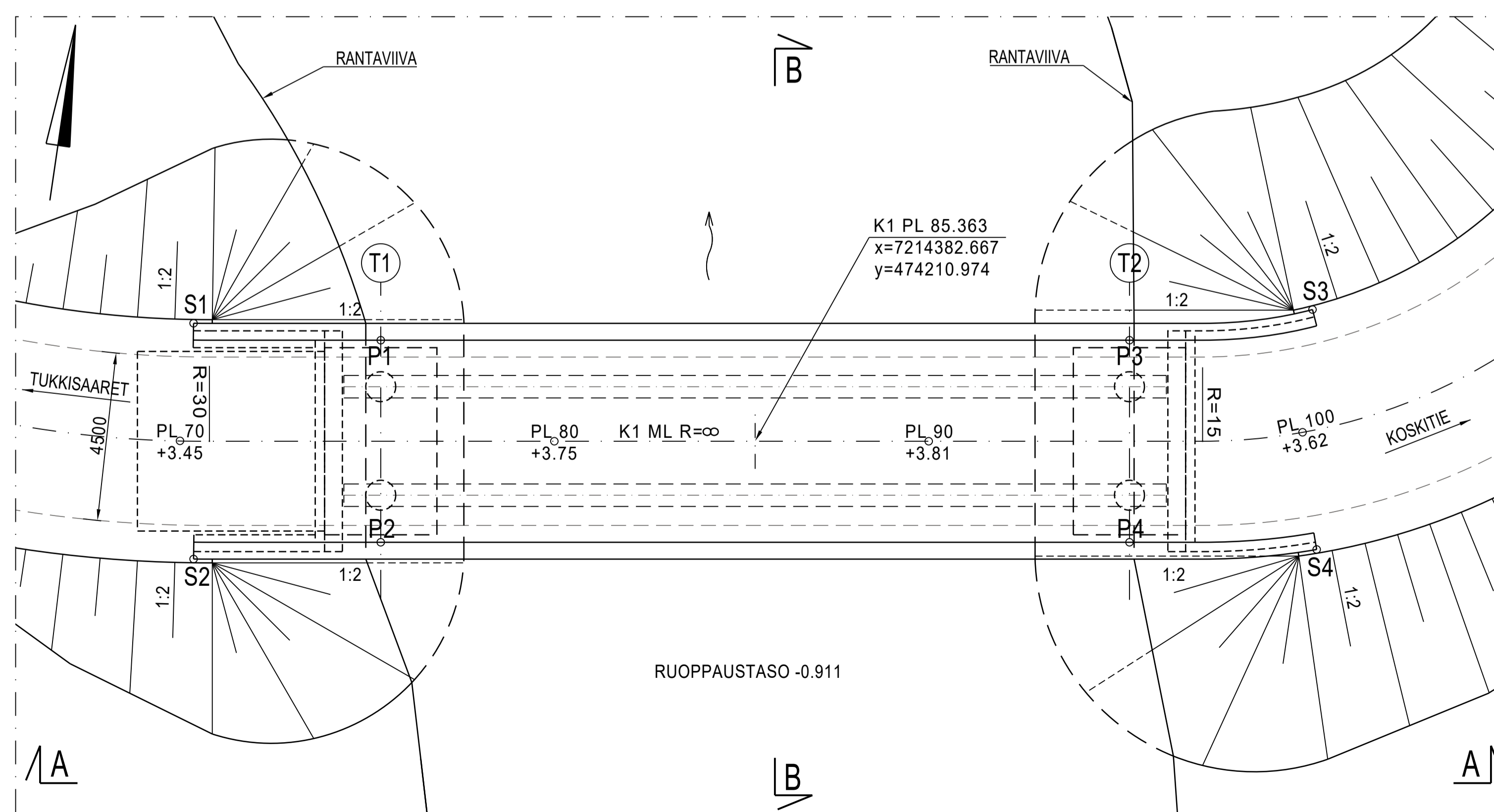
TASOPIIRUSTUS 1:100
