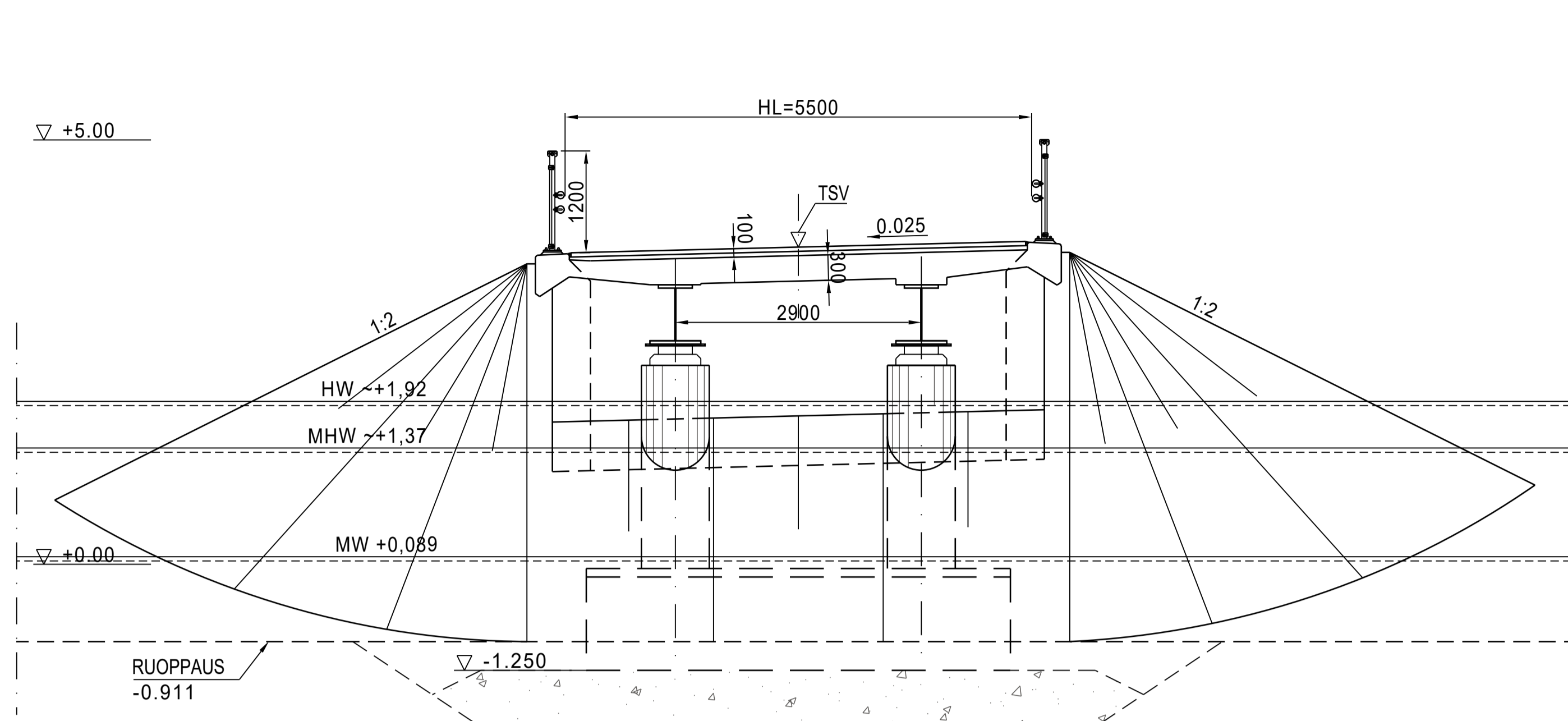
B-B 1:50
