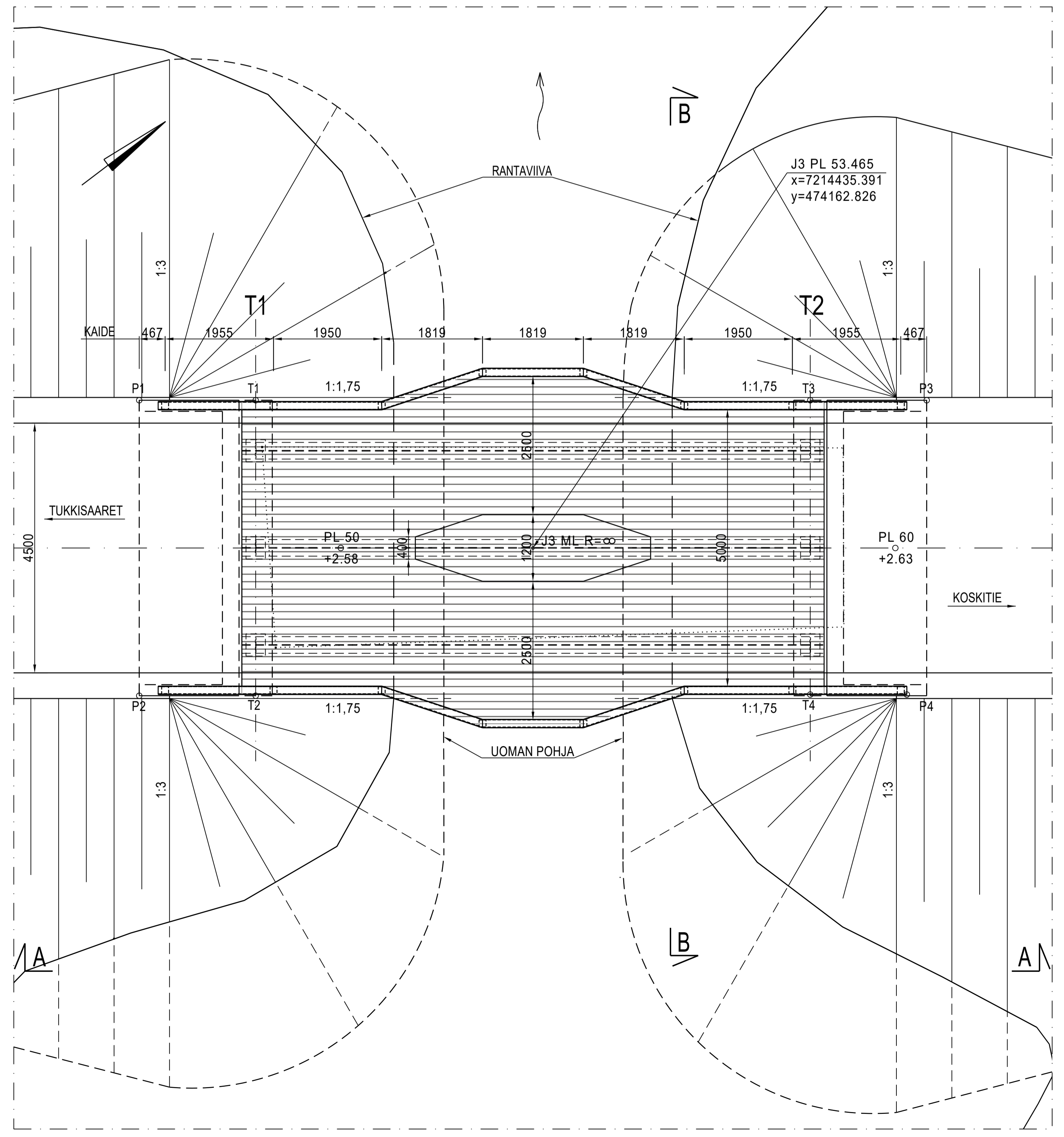
TASOPIIRUSTUS 1:50
